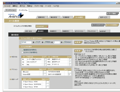
メール設定—基本設定画面
